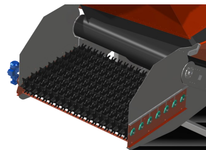
ÉBRANCHEUR ÉTOILÉ DIRECTEMENT EN SORTIE DE TRÉMIE (SANS TAPIS TRANSVERSAL)
